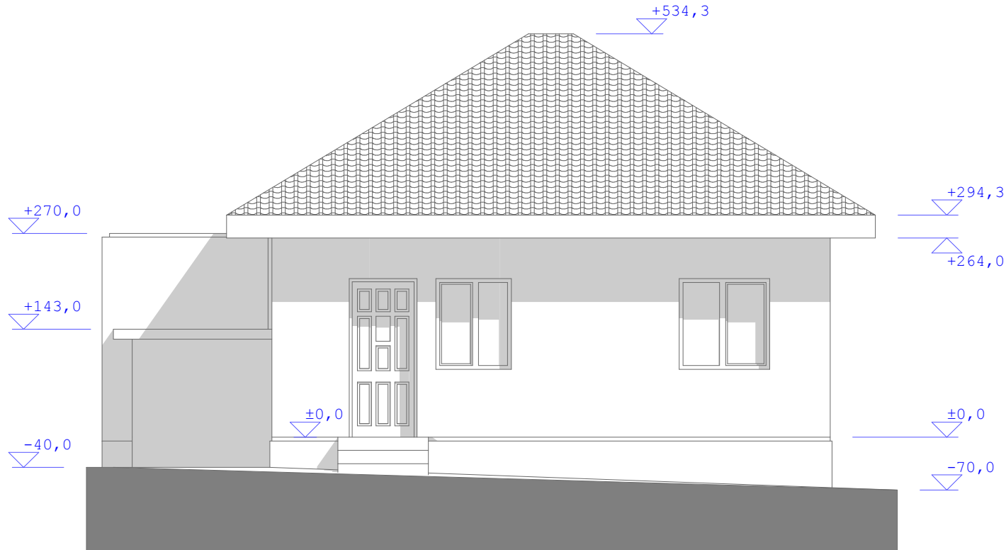
FAȚADA SUD-VEST - SITUAȚIA EXISTENTĂ 1:70
